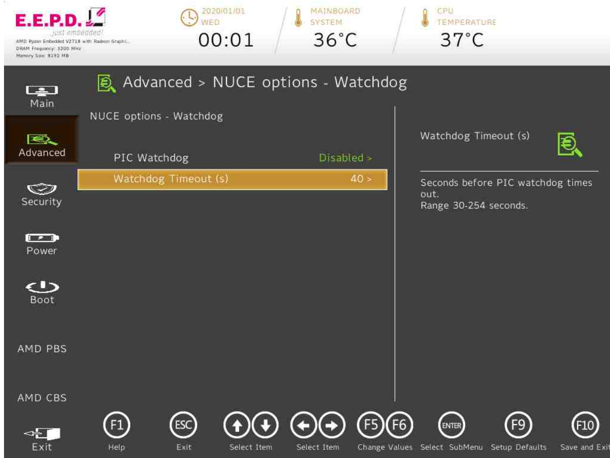
Fig. 29: NUCE options
